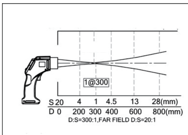
Pro1300L-LC2 Pro1300L-HC2
