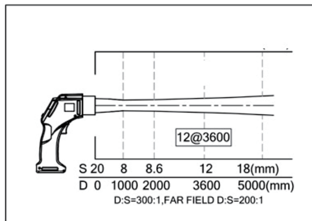
Pro1300L-LS Pro1300L-HS
