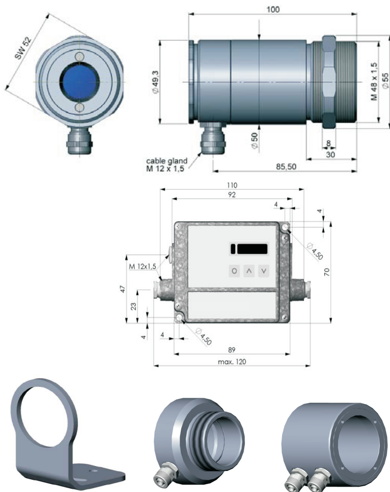
外形寸法図
